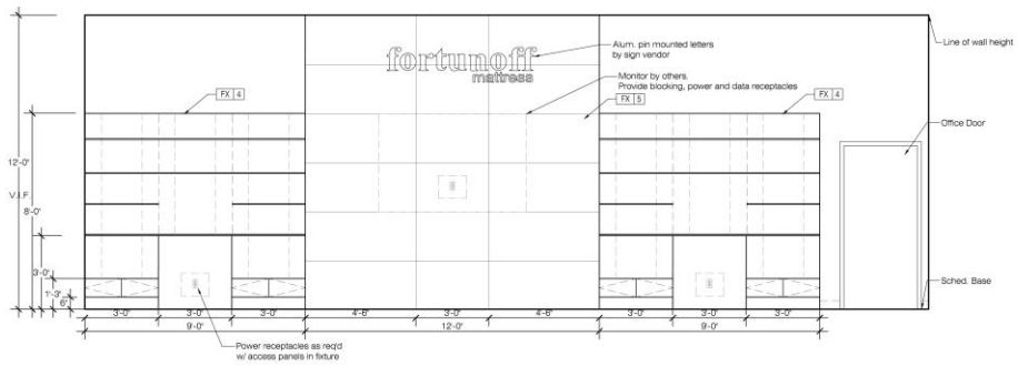
2 ELEVATION 1 SCALE: 3/8" = 1'-0"
