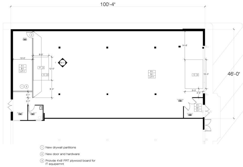
1 FLOOR PLAN SCALE: 1/8" = 1'-0"
